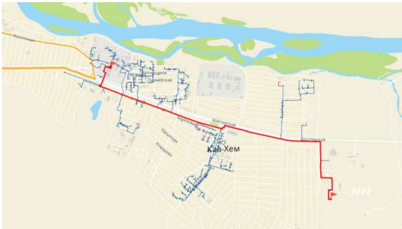
Рисунок 2.13 – Путь теплоносителя по направлению от КТЭЦ до потребителя «Общеобразовательная школа»
