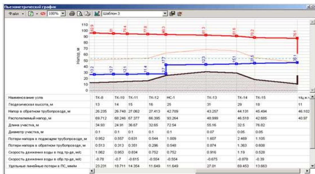
Рисунок 2.18 - Пьезометрический график
